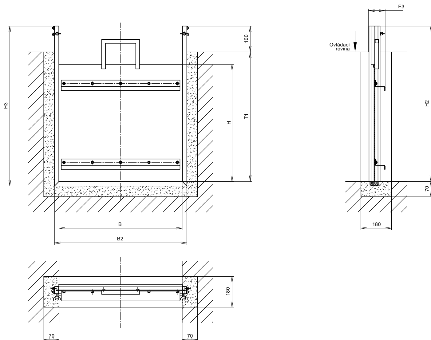
Ruční hradítko
