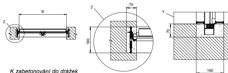
K zabetonování do drážek
